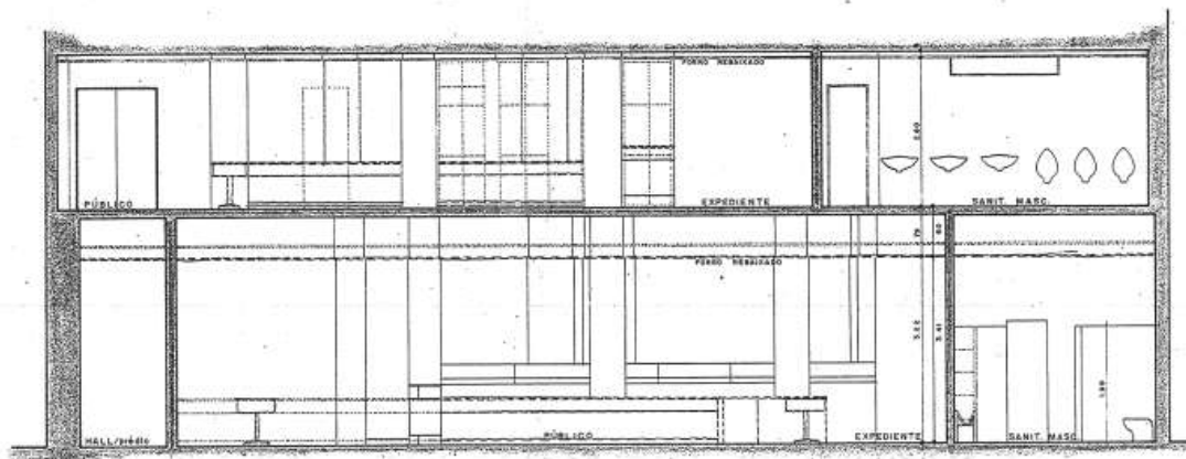
CORTE C.D
